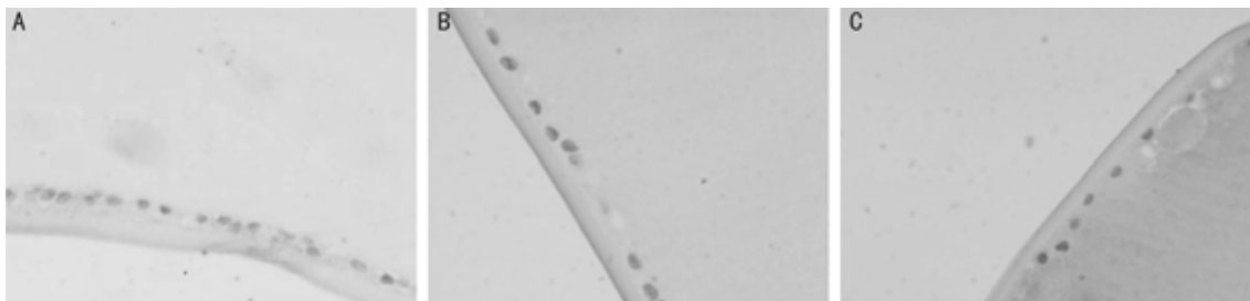
图2 培养 LEC 凋亡(TUNEL ×400) A:空白对照组;B:Dex 组;C:EGCG 组。
