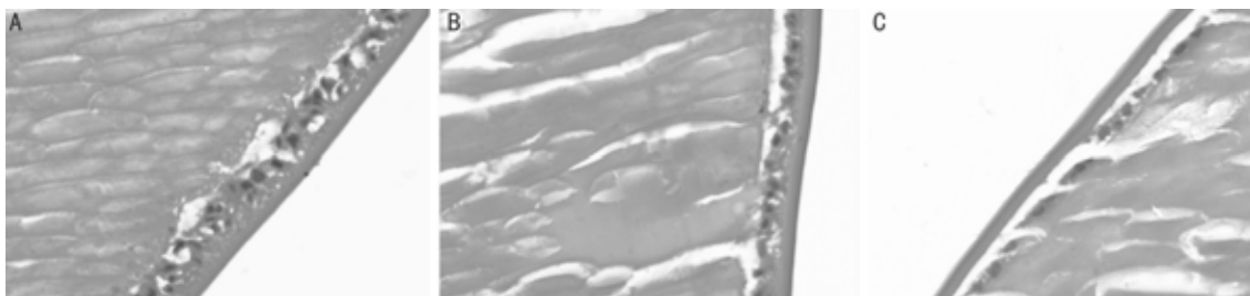
图1 培养晶状体上皮细胞(HE ×400) A:空白对照组;B:Dex 模型组;C:EGCG 组。
